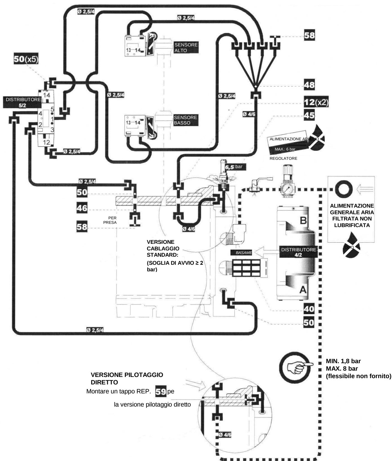
Schema pneumatico - Motore 3000
